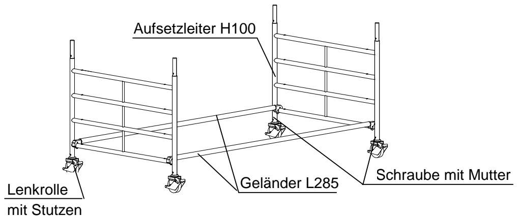
Bild 2: Grundeinheit ohne Fahrbalken, SH 2.10 m
