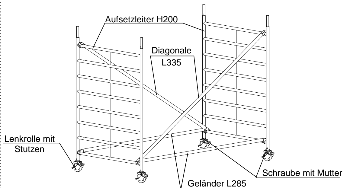
Bild 3: Grundeinheit ohne Fahrbalken, Standhöhe 3.10 m
