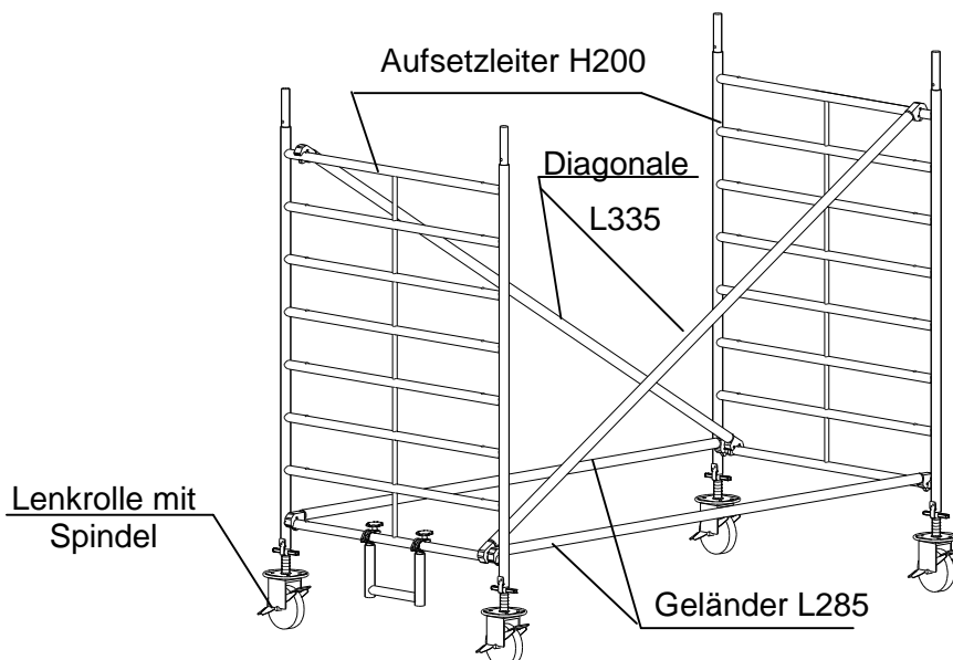
Bild 5: Grundeinheit ohne Fahrbalken, Standhöhe 5.50 m
