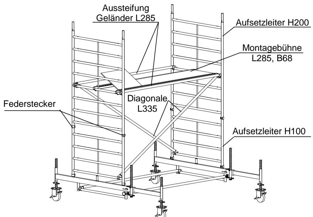
Bild 9: Montagebühne Standhöhe 2.60 m
