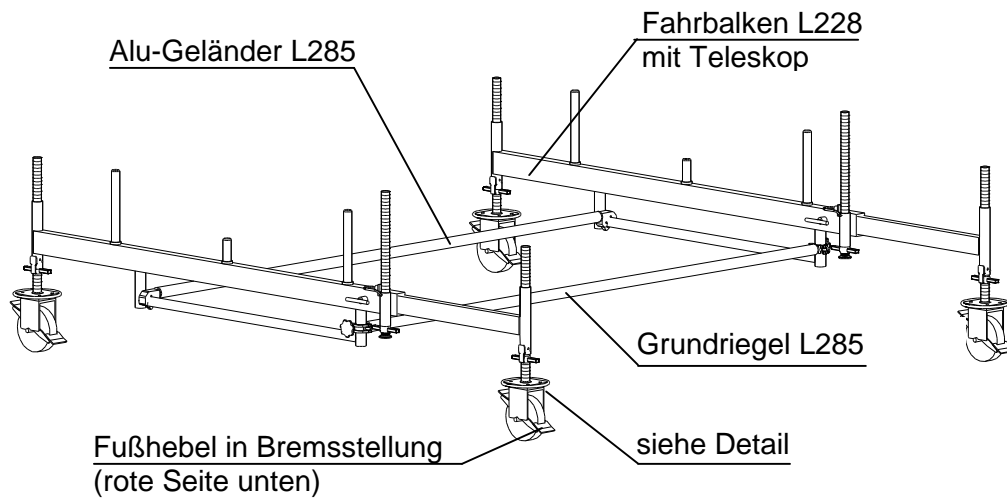
Bild 1: Fahrwerk mit Teleskop-Fahrbalken L228
