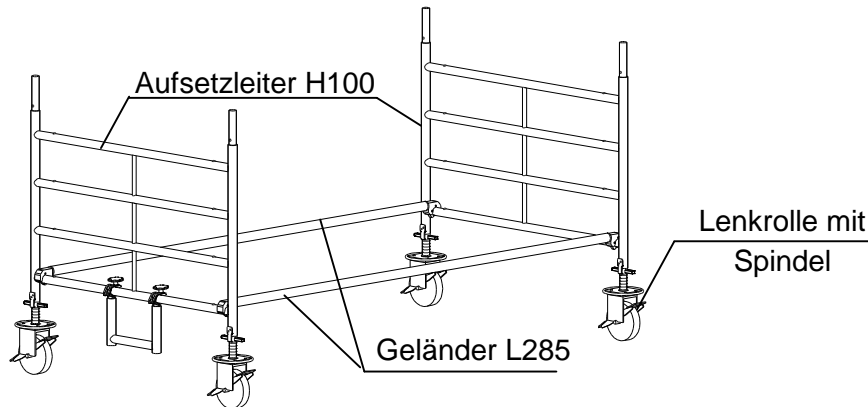
Bild 4: Grundeinheit ohne Fahrbalken, Standhöhe 4.50 m
