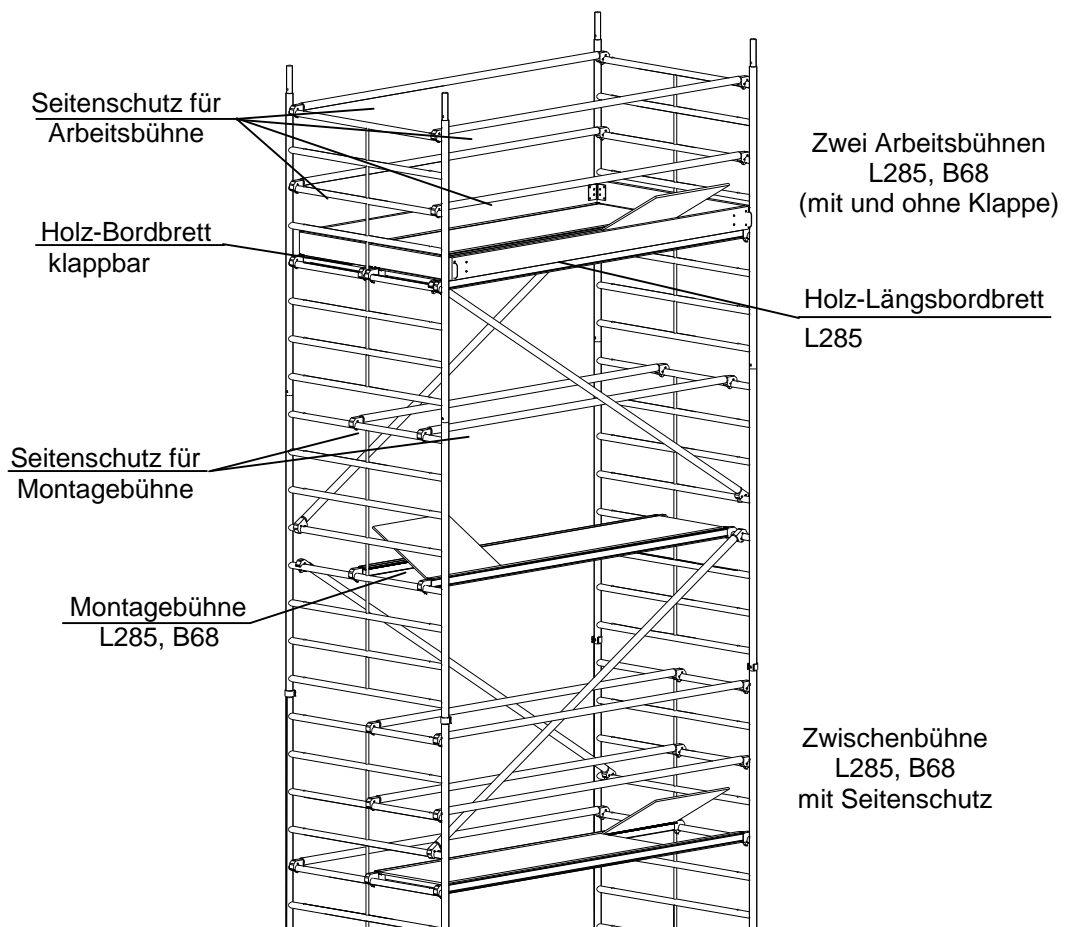
Bild 13: Oberer Gerüstbereich mit Arbeitsbühne
